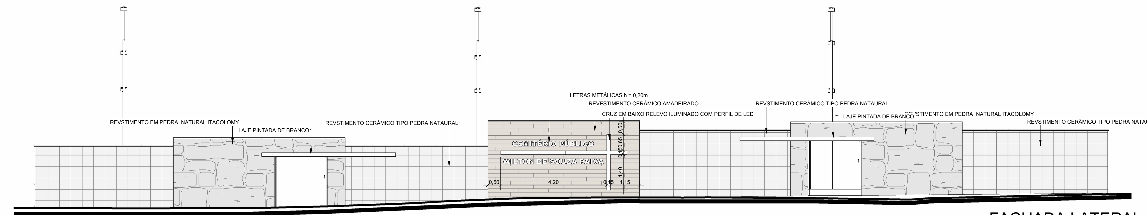
1 FACHADA LATERAL 1 : 75
